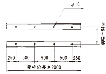
アンカーボルト取付位置
