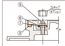
密閉形 (ボルトロック式)
