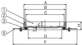
ボルト固定部詳細
