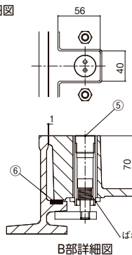
B部詳細図
