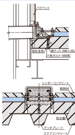
納まり図(参考)
