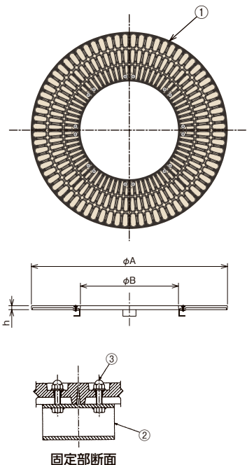
固定部断面
