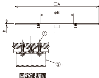
固定部断面
