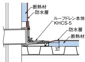
KHCS-5 納まり図
