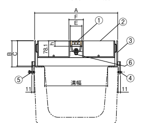
※黒色仕上 U6DJ…K / U10DJ…K 化粧蓋・受枠:ケンポージック
