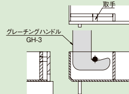
取手部詳細
