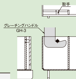
スキマ6mm 取手部詳細
