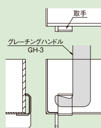
スキマ9.5mm 取手部詳細
