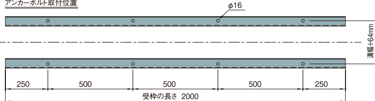
アンカーボルト取付位置
