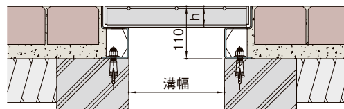
アンカーボルト取付位置
