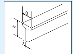
TP-GM ベアリングバー詳細図
