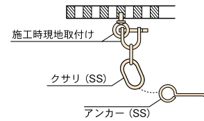
盗難防止用クサリ取付詳細
