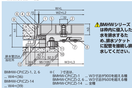
■断面詳細・納まり図
