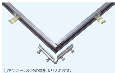
①アンカーは外枠の端部より入れます。
