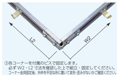
②平坦な所に外枠4本を置き、コーナー金具を入れます。このとき、コーナー金具の方向に注意してください。
