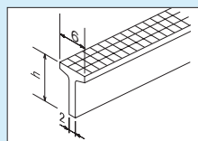
TX-GM ベアリングバー詳細図
