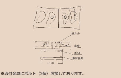
取付金具組立図
