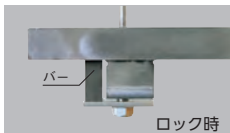
② 固定金具が受枠側のバーの下に潜り込んでいる事を確認しドライバーでねじ込みます。
