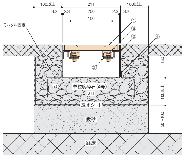
ベアリングバー詳細図
