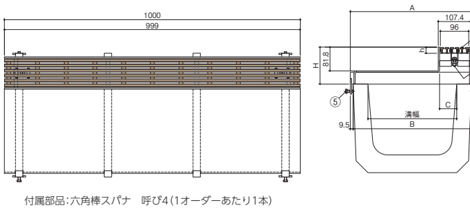
付属部品:六角棒スパナ 呼び4 (1オーダーあたり1本)
