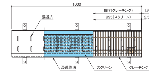
枠端部 (エンドプレート付)
