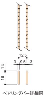
ベアリングバー詳細図
