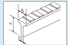
TW-GM ベアリングバー詳細図
