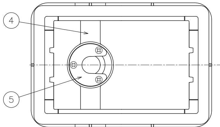
蓋なし平面図
