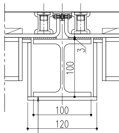
受梁部断面詳細図 S=1/4
