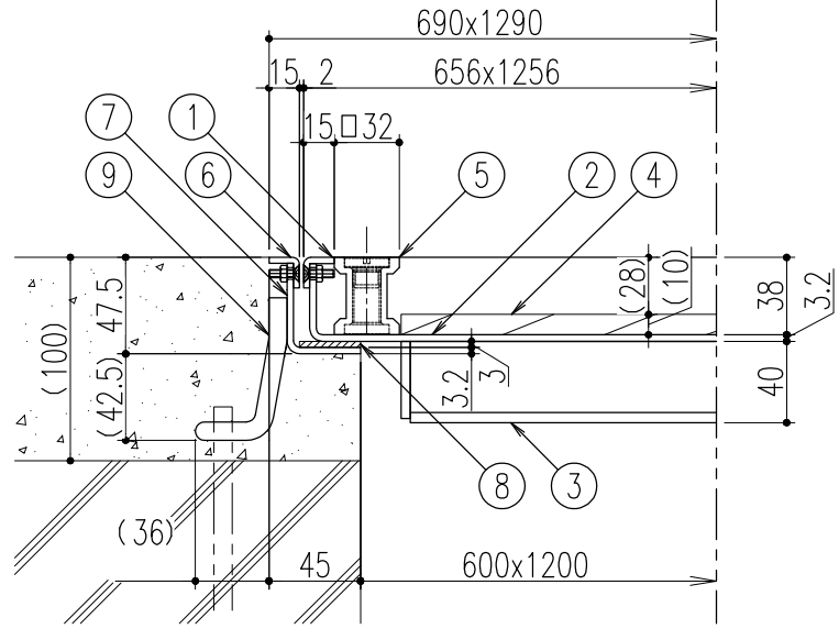
断面詳細図 S=1/4
