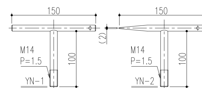
Yハンドル 材質：銅製 / 表面处理：ユニクロメッキ
