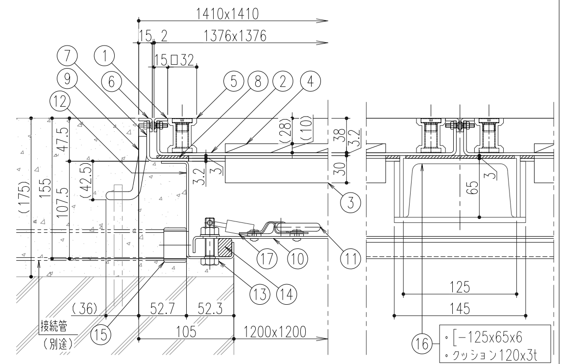
断面詳細図 S=1/4
