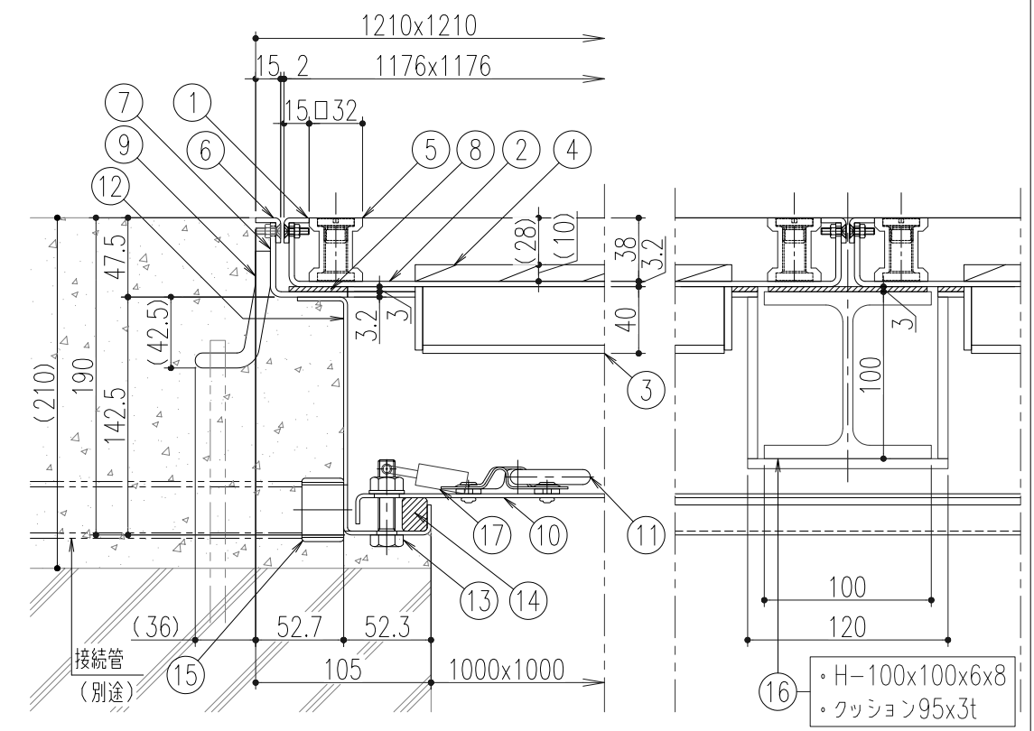
断面詳細図 S=1/4
