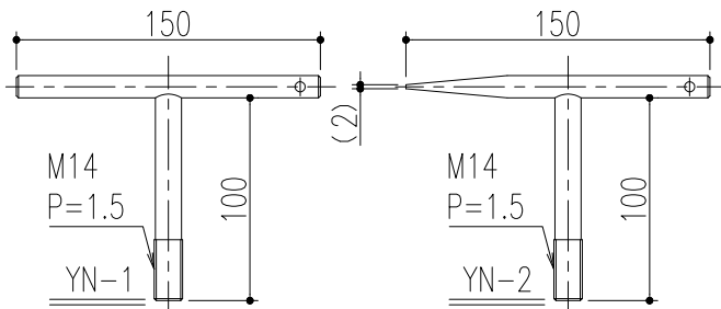
Yハンドル 材質：鋼製 / 表面处理：ユニクロメッキ
