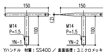
Yハンドル 材質: SS400 / 表面処理: ニクロメッキ
