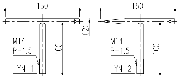
Yハンドル 材質：銅製 / 表面処理：ユニクロメッキ
