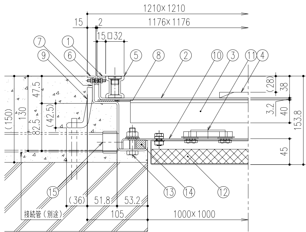
断面詳細図 S=1/4
