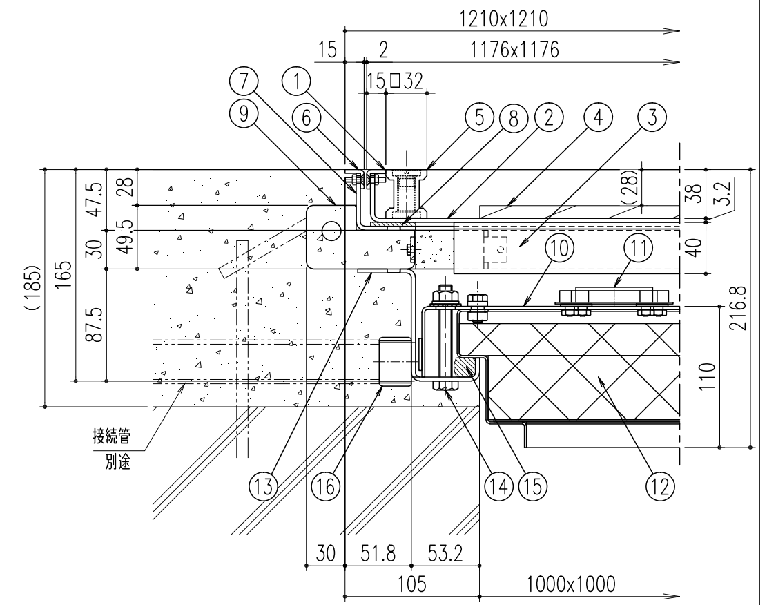
断面詳細図 S=1/4
