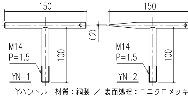
Yハンドル 材質：銅製 / 表面処理：ユニクロメッキ
