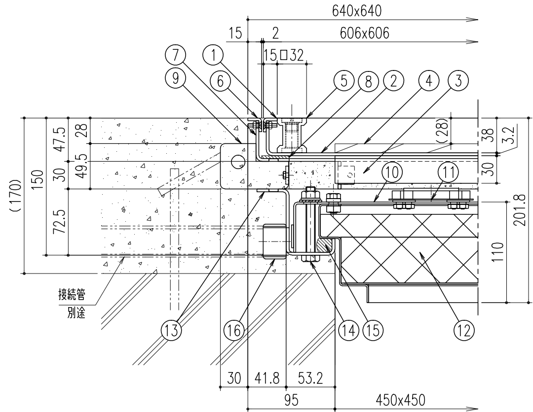
断面詳細図 S=1/4
