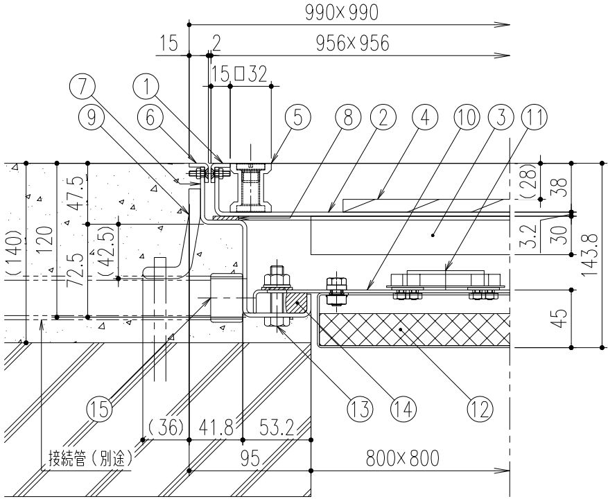
断面詳細図 S=1/4
