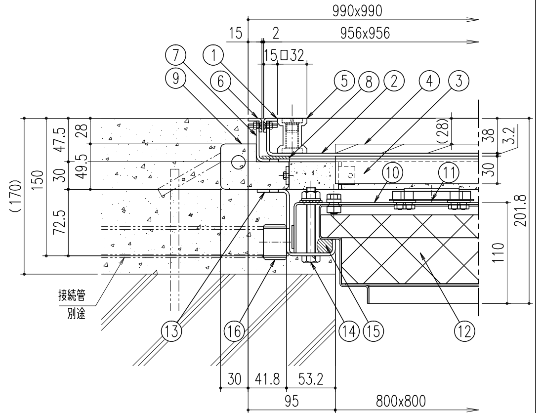
断面詳細図 S=1/4
