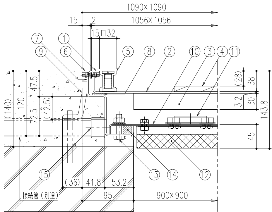
断面詳細図 S=1/4
