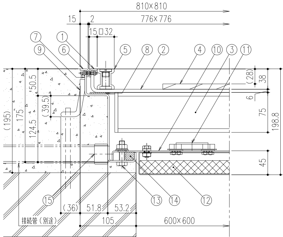
断面詳細図 S=1/4
