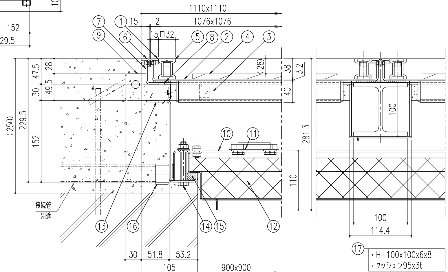
断面詳細図 S=1/4
