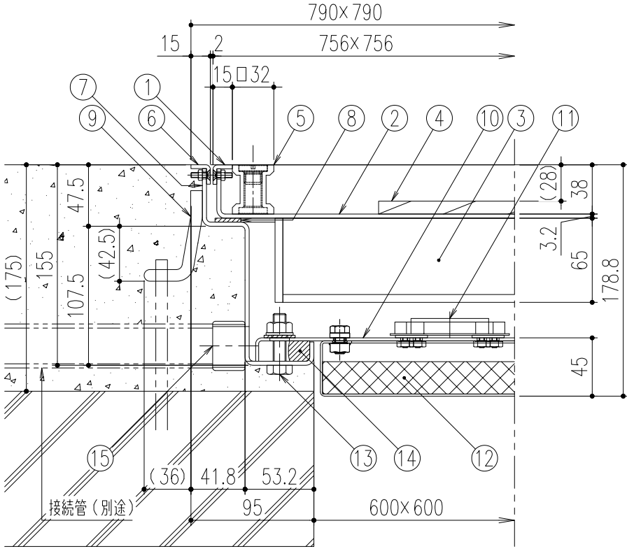
断面詳細図 S=1/4
