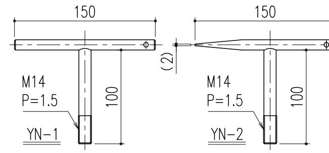
Yハンドル 材質：鋼製 / 表面処理：ユニクロメッキ
