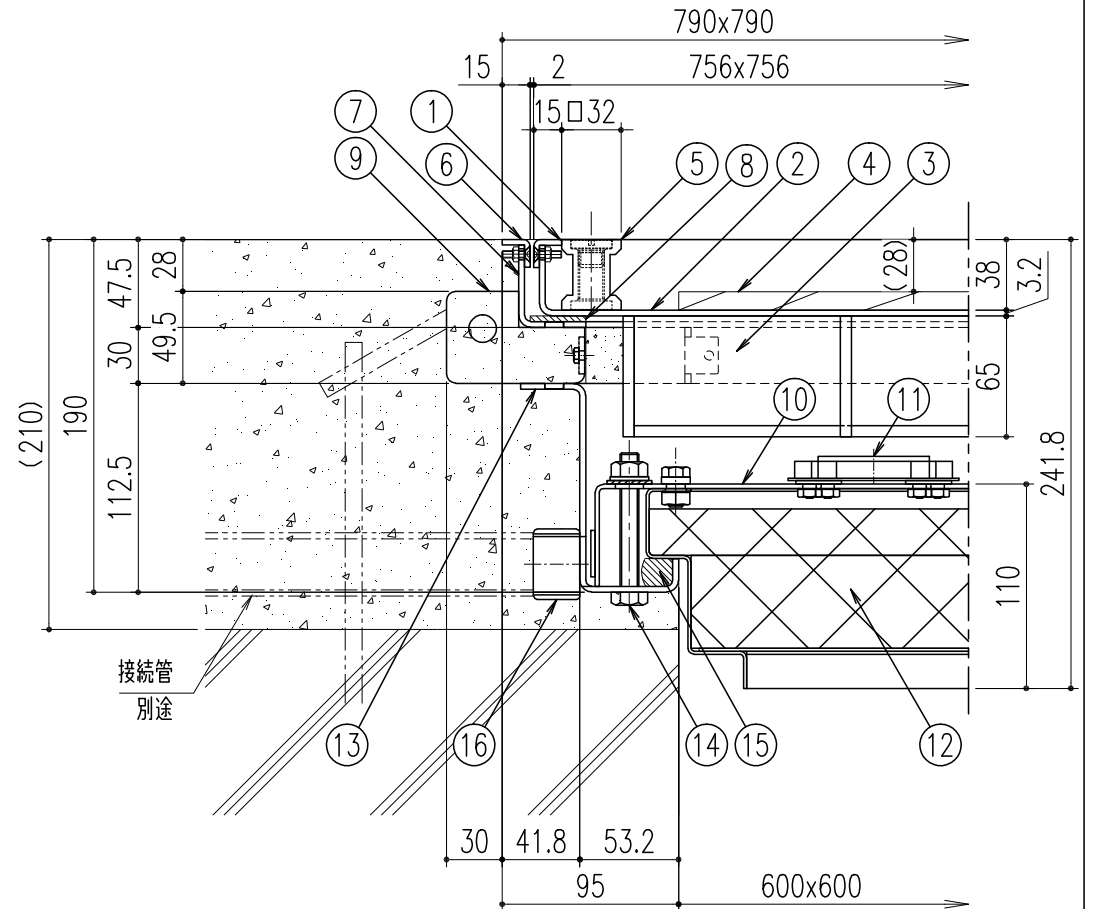
断面詳細図 S=1/4
