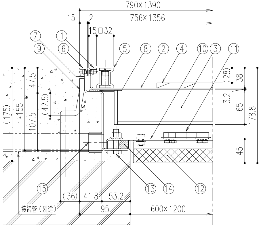
断面詳細図 S=1/4
