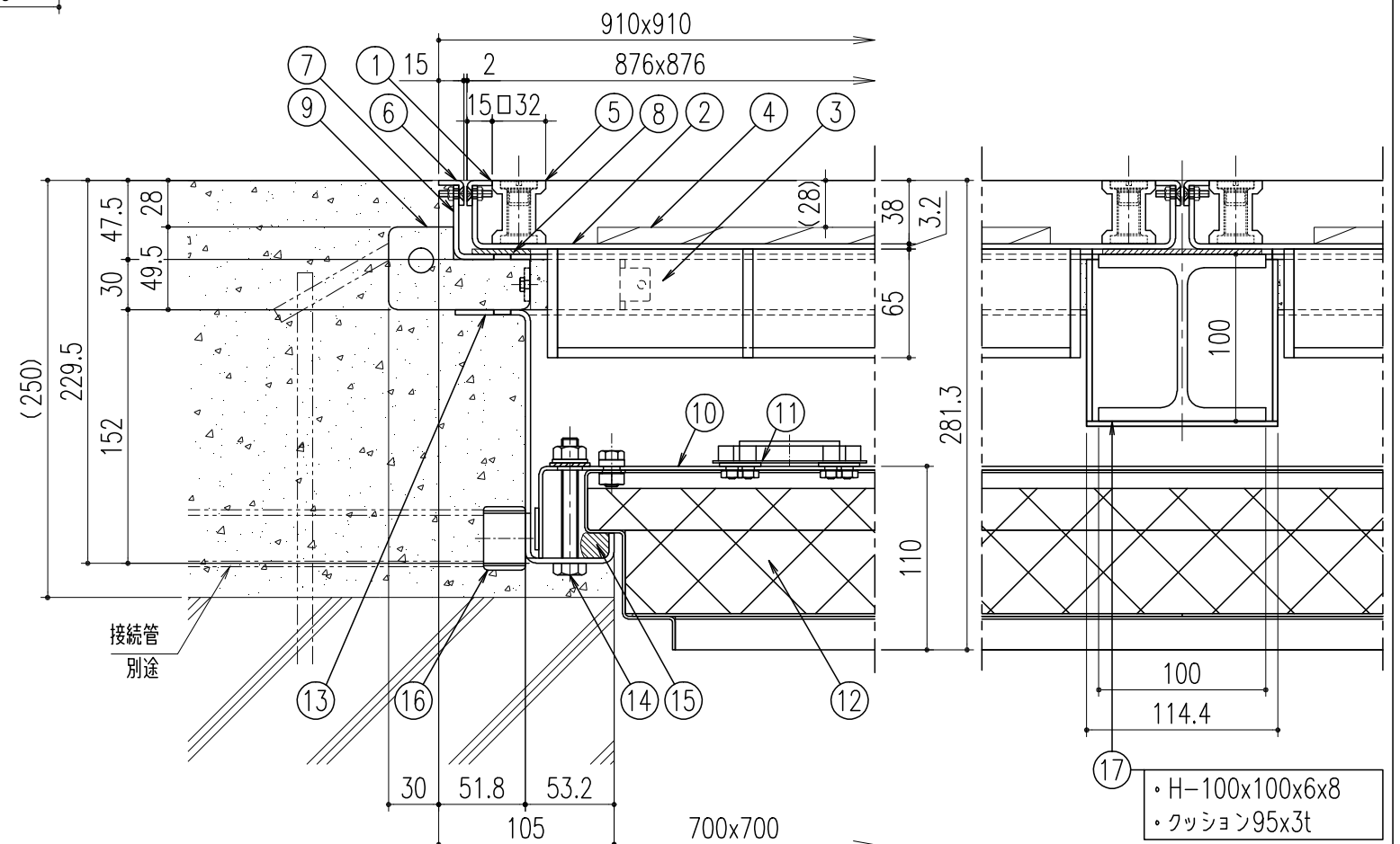
断面詳細図 S=1/4
