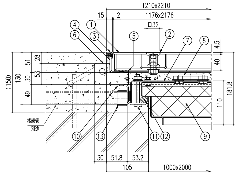
断面詳細図 S=1/4
