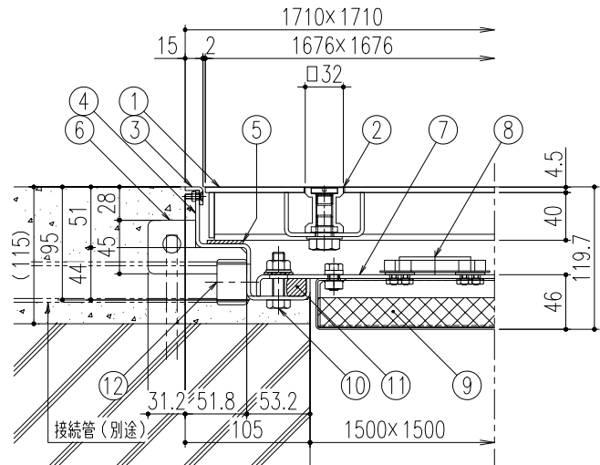
断面詳細図 S=1/4
