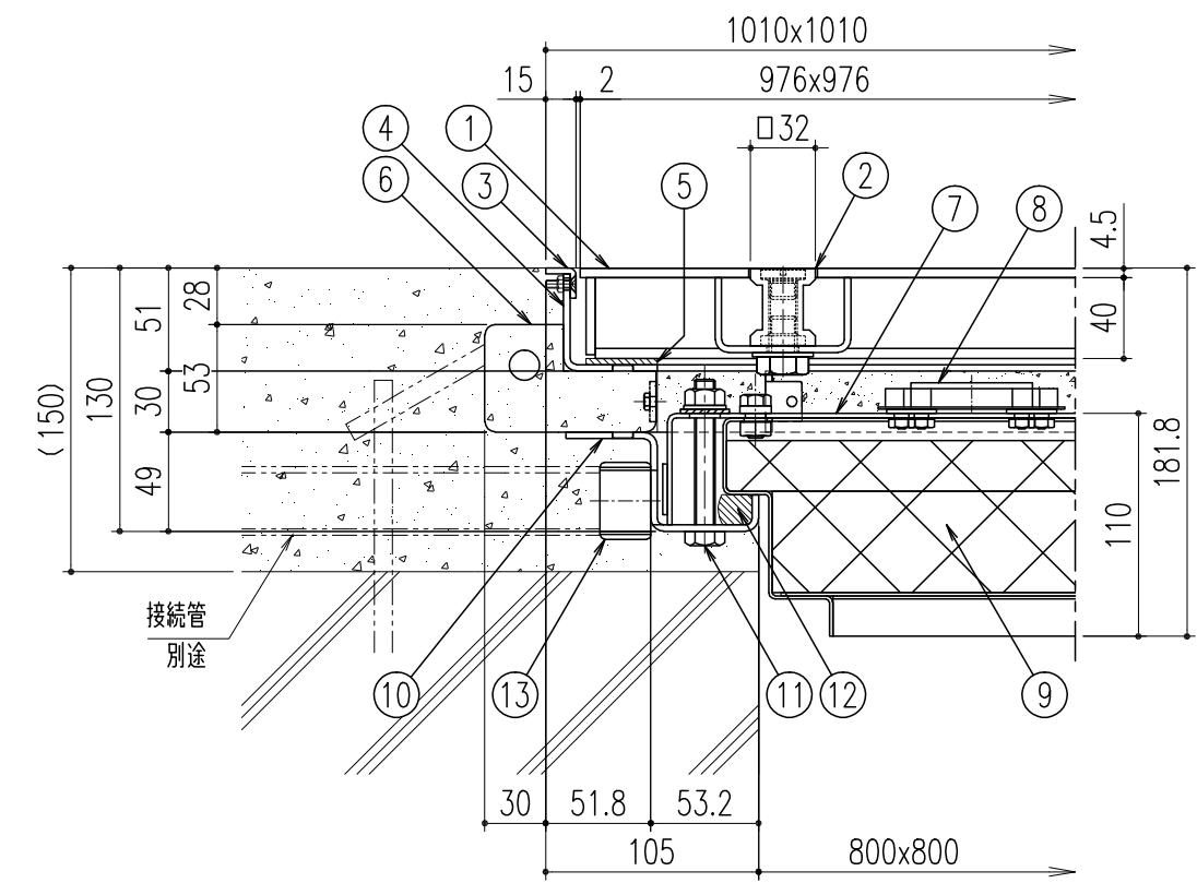
断面詳細図 S=1/4
