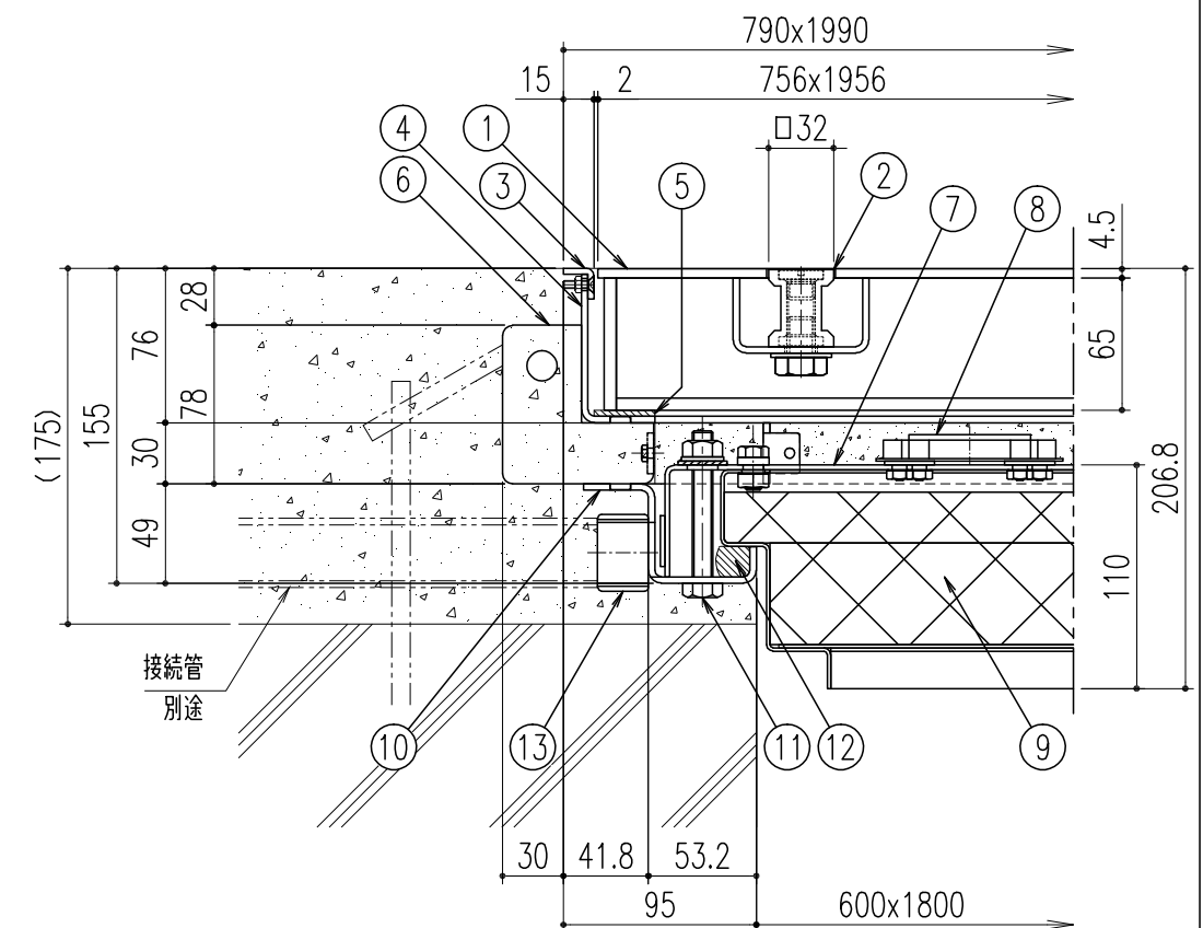
断面詳細図 S=1/4
