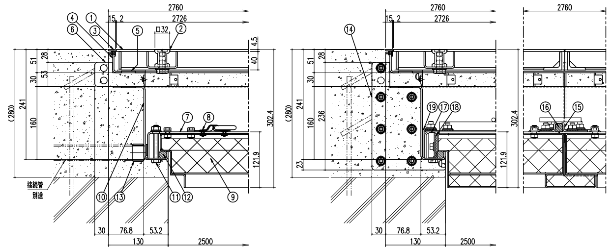
断面(連結部)詳細図 S=1/4
