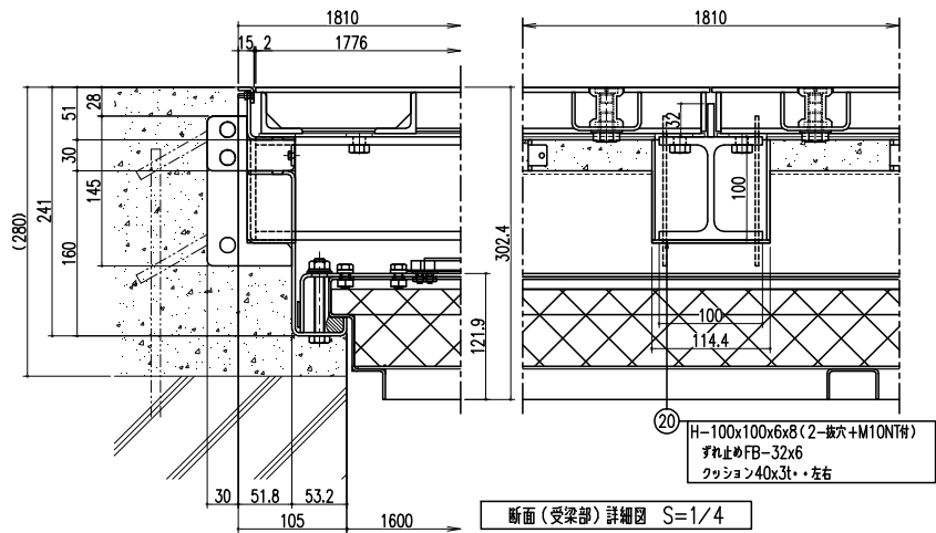
断面詳細図 S=1/4
