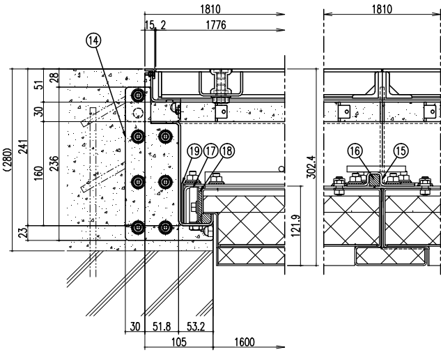
断面(連結部)詳細図 S=1/4
