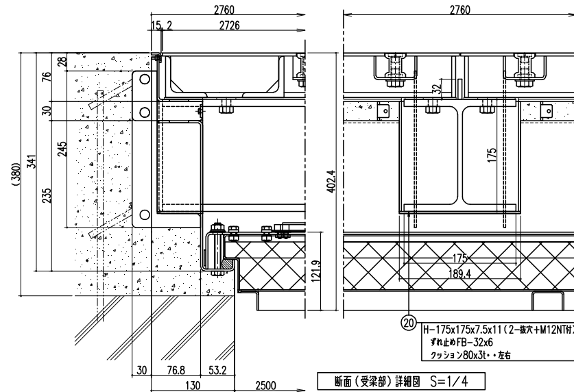
断面(受梁部)詳細図 S=1/4
