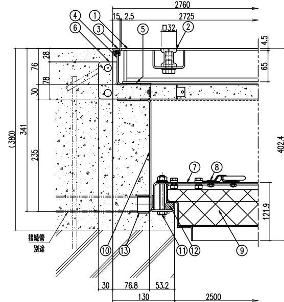
断面詳細図 S=1/4
