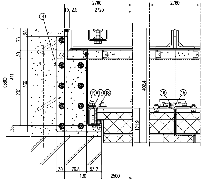
断面（連結部）詳細図 S=1/4
