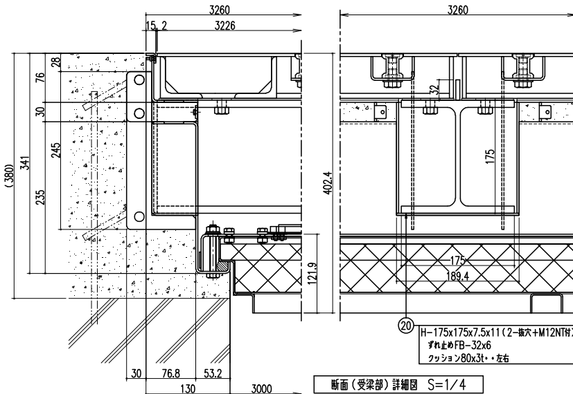
断面(受梁部)詳細図 S=1/4
