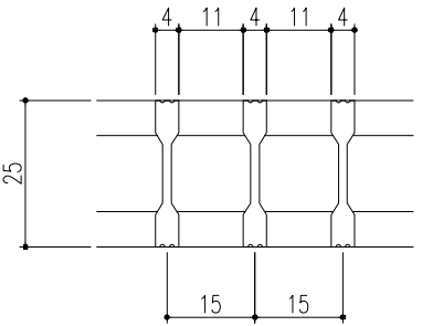
ベアリングバー断面詳細図
