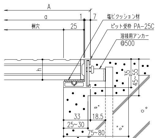
断面詳細図 S=1/2
