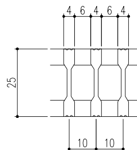
ベアリングバー断面詳細図
