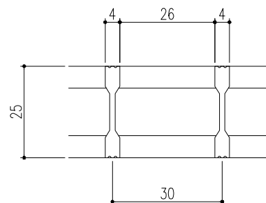
ベアリングバー断面詳細図
