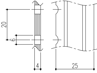
ベアリングバー詳細図
