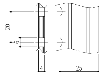
ベアリングバー詳細図
