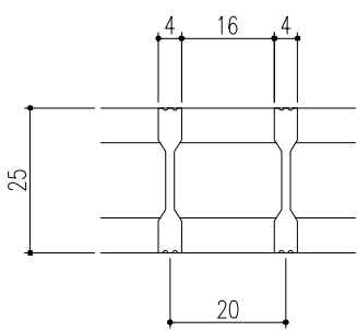
ベアリングバー断面詳細図
